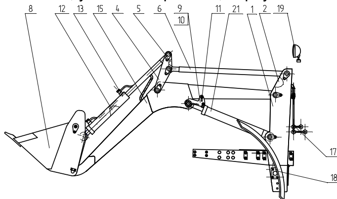
1-2 – порталы; 4-5 – рычаги; 6 – тяги; 8 – ковш; 9-10-упоры; 11-стопор; 12-13-гидроцилиндры 15-стрела; 17-гидросистема; 18-установка крыльев; 19-переустановка фар; 21-гидроцилиндры Рисунок 2.3 – Погрузочное оборудование
