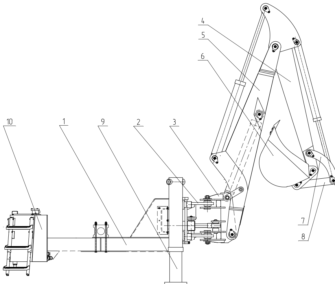
1 рама; 2 – подвижная каретка; 3 – колонка; 4 – рукоять; 5-стрела; 6-ковш; 7-рычаги; 8-рычаг; 9-опоры; 10-гидробак Рисунок 2.2 – Экскаваторное оборудование
