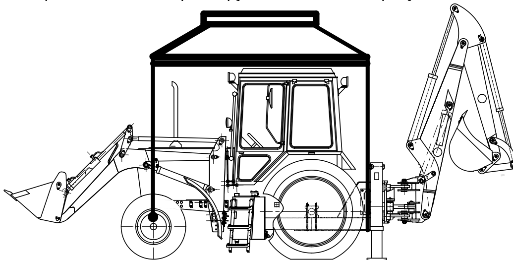
Рис.7.1-Схема строповки
