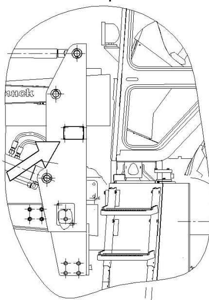
Рис.1.2. Местоположение маркировочной таблички
