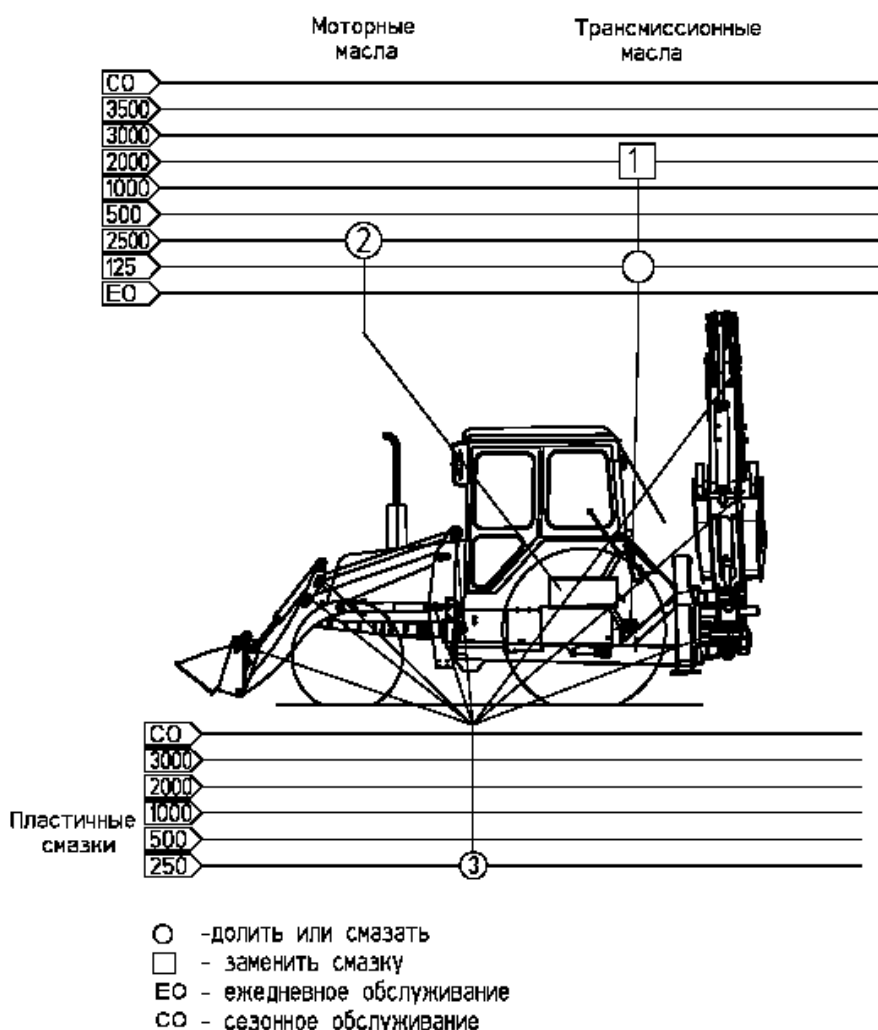
Рисунок 4.1 – Схема смазки
