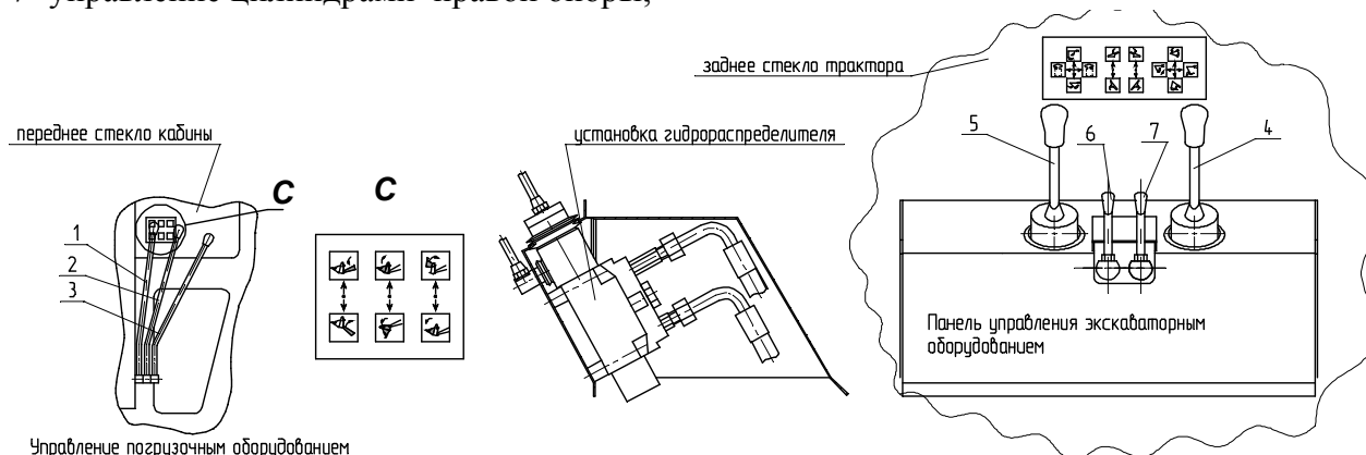
Рисунок 2.1 – Расположение рычагов и педалей управления
