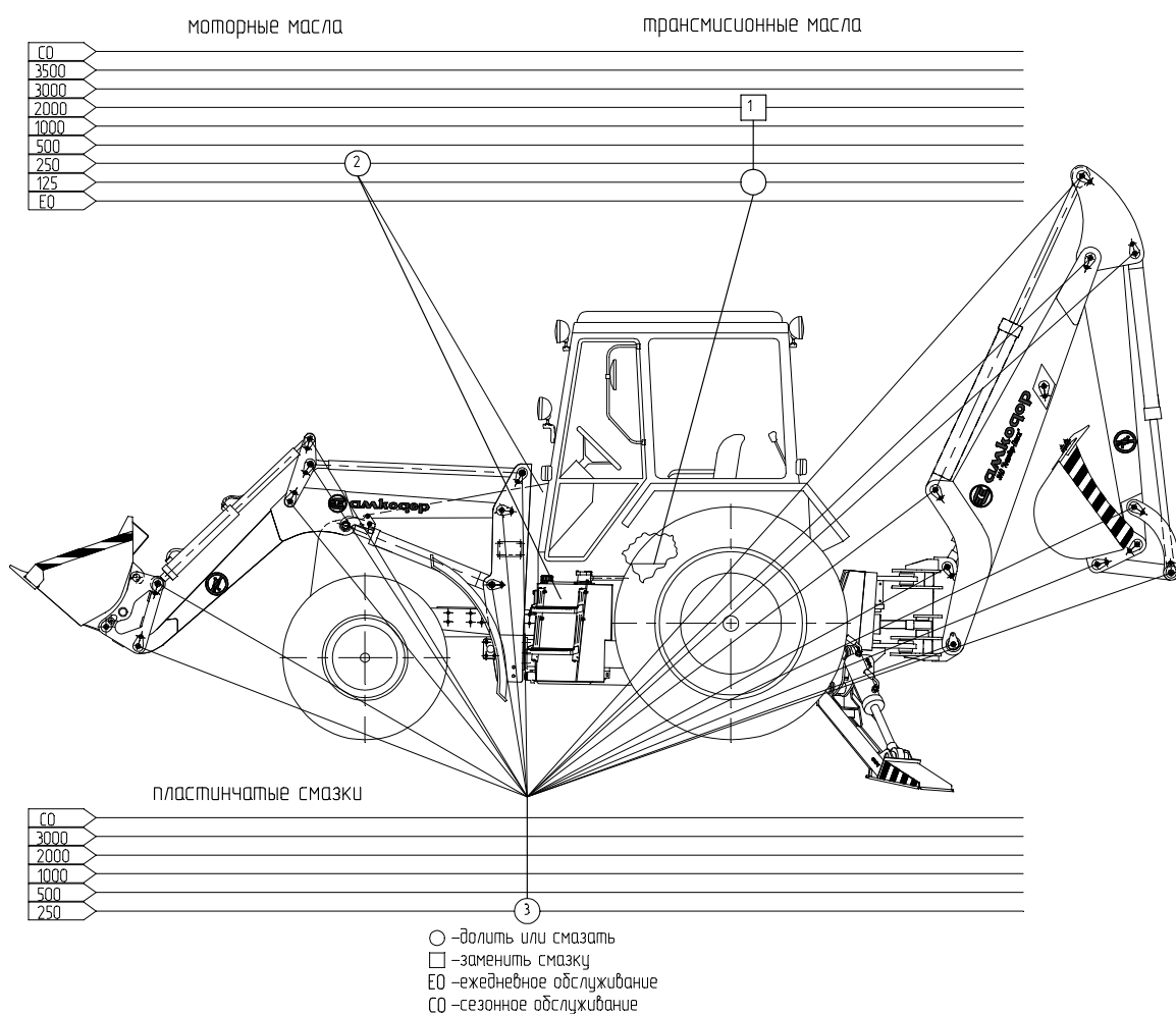
Рисунок 4.1 – Схема смазки
