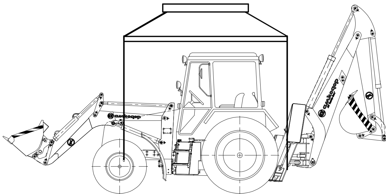
Рис.7.1-Схема строповки
