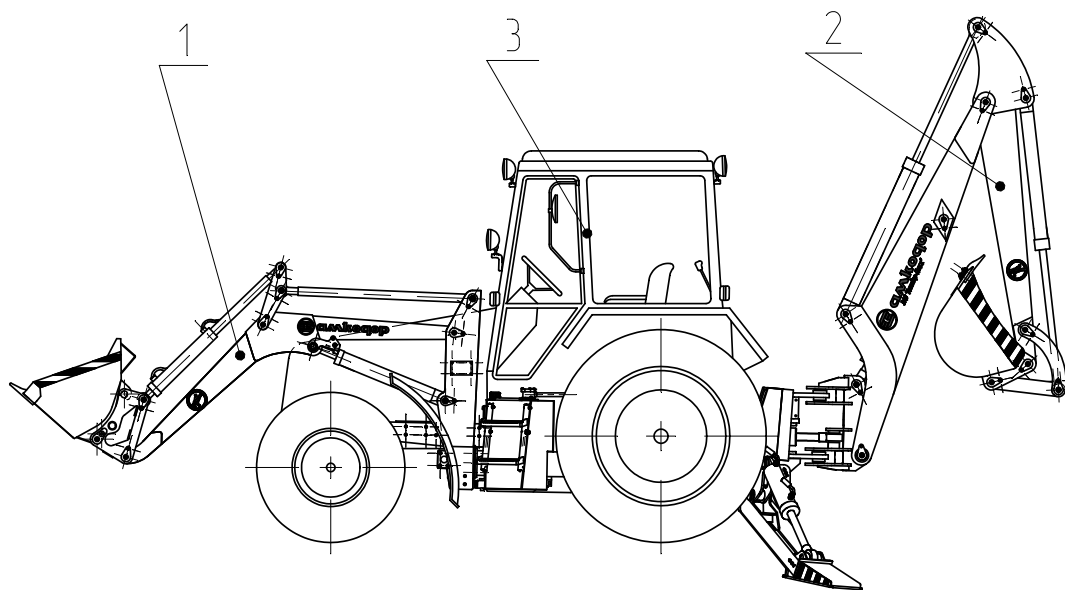
1 – погрузочное оборудование; 2 – экскаваторное оборудование; 3 – базовая машина
